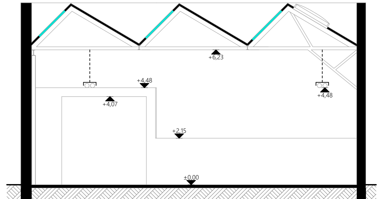
Coupe 2
