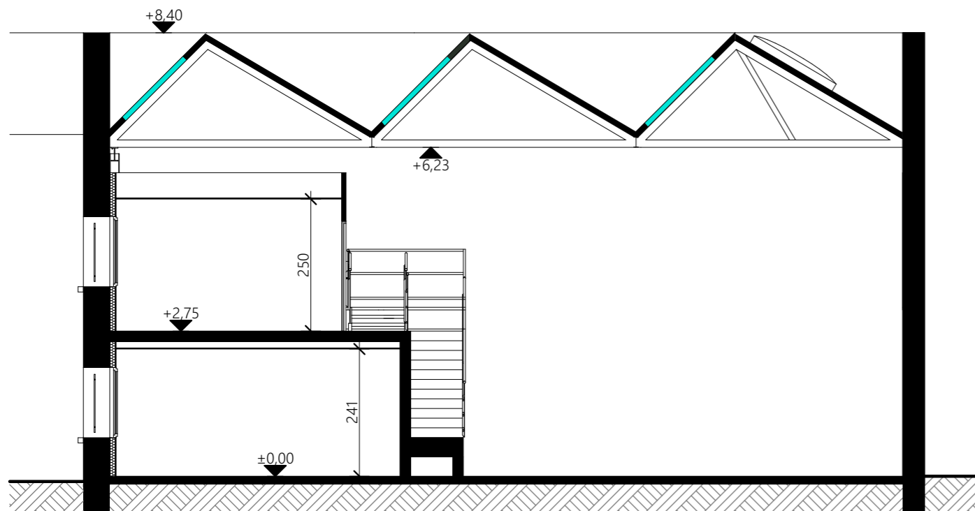
Coupe 1
